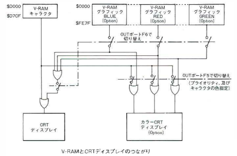
V-RAMとCRTディスプレイのつながり
