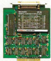
GP-IBインターフェイスカード MZ-8BI04 標準価格 45,000円
